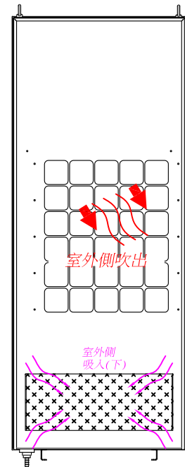
KA-302SAL 後視圖 Frank G0913
