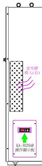
KA-302SAR 右側視圖
